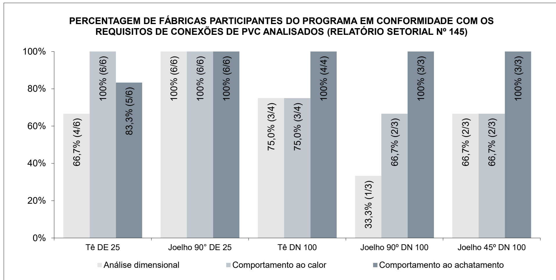
Figura 13 - Conexões de PVC - Fábricas participantes em conformidade com os requisitos analisados pelo Programa Setorial da Qualidade – Relatório Setorial nº 145
