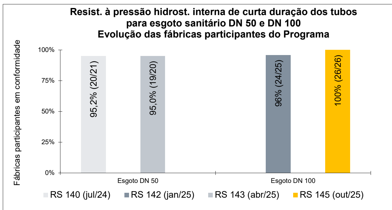
Figura 5 - Verificação da resistência à pressão hidrostática interna de curta duração dos tubos para esgoto sanitário DN 50 e DN 100
