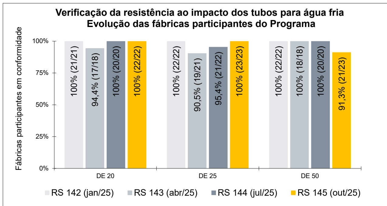
Figura 6 - Verificação da resistência ao impacto a 0°C dos tubos para água fria DE 20, DE 25 e DE 50
