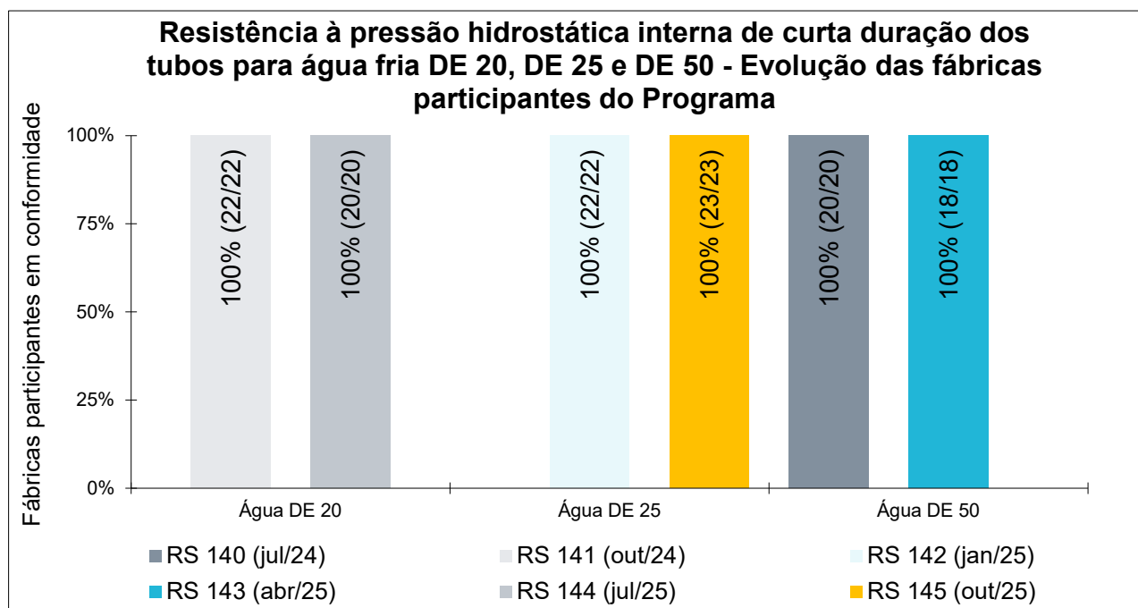
Figura 4 - Verificação da resistência à pressão hidrostática interna de curta duração dos tubos para água fria DE 20, DE 25 e DE 50
