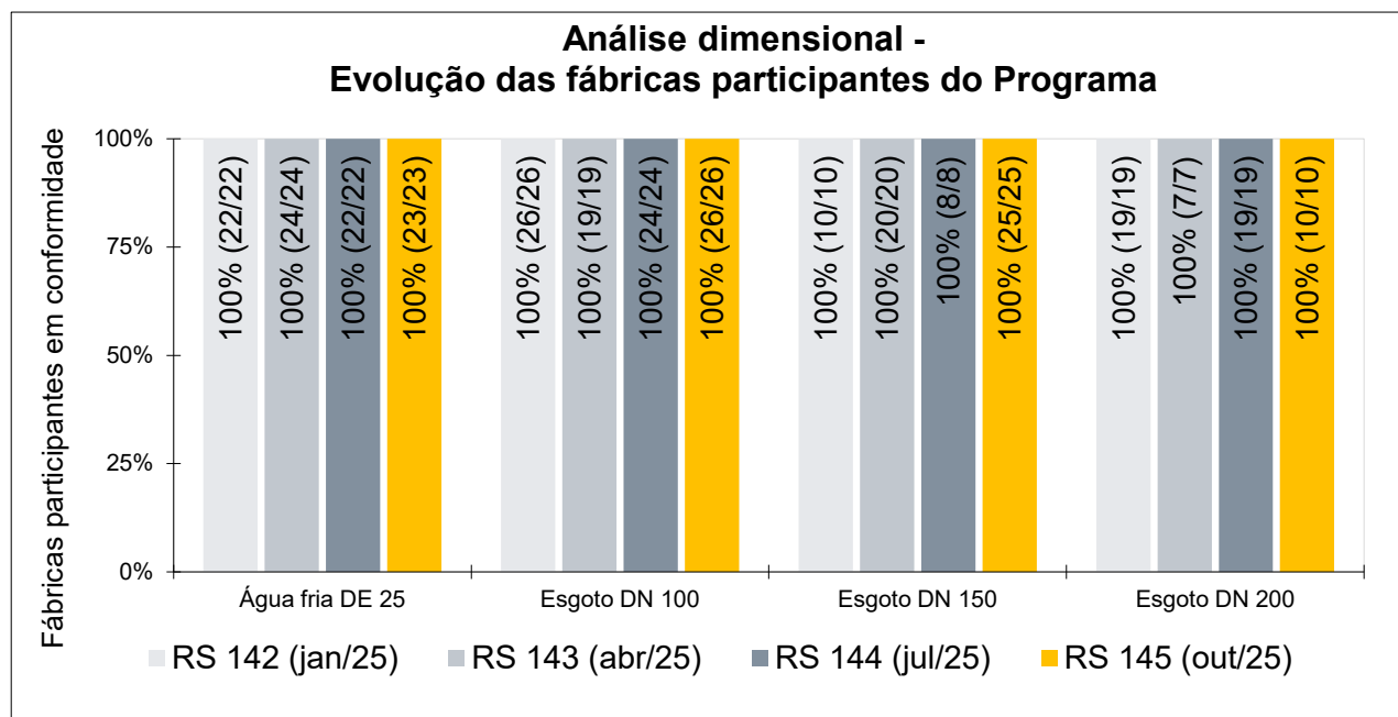
Figura 2 - Análise dimensional dos tubos para água fria DE 25 e tubos para esgoto sanitário SN DN 100, DN 150 e DN 200
