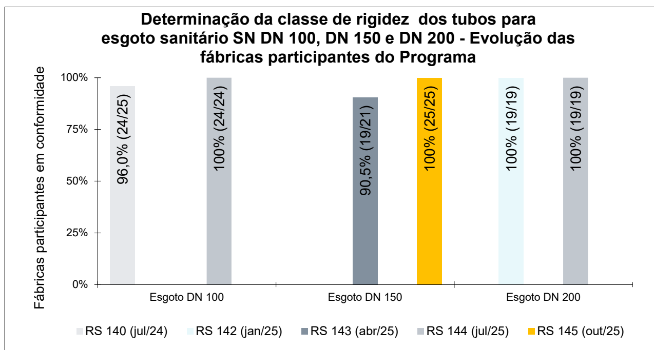
Figura 7 - Verificação da classe de rigidez dos tubos para esgoto sanitário SN DN 100, DN 150 e DN 200
