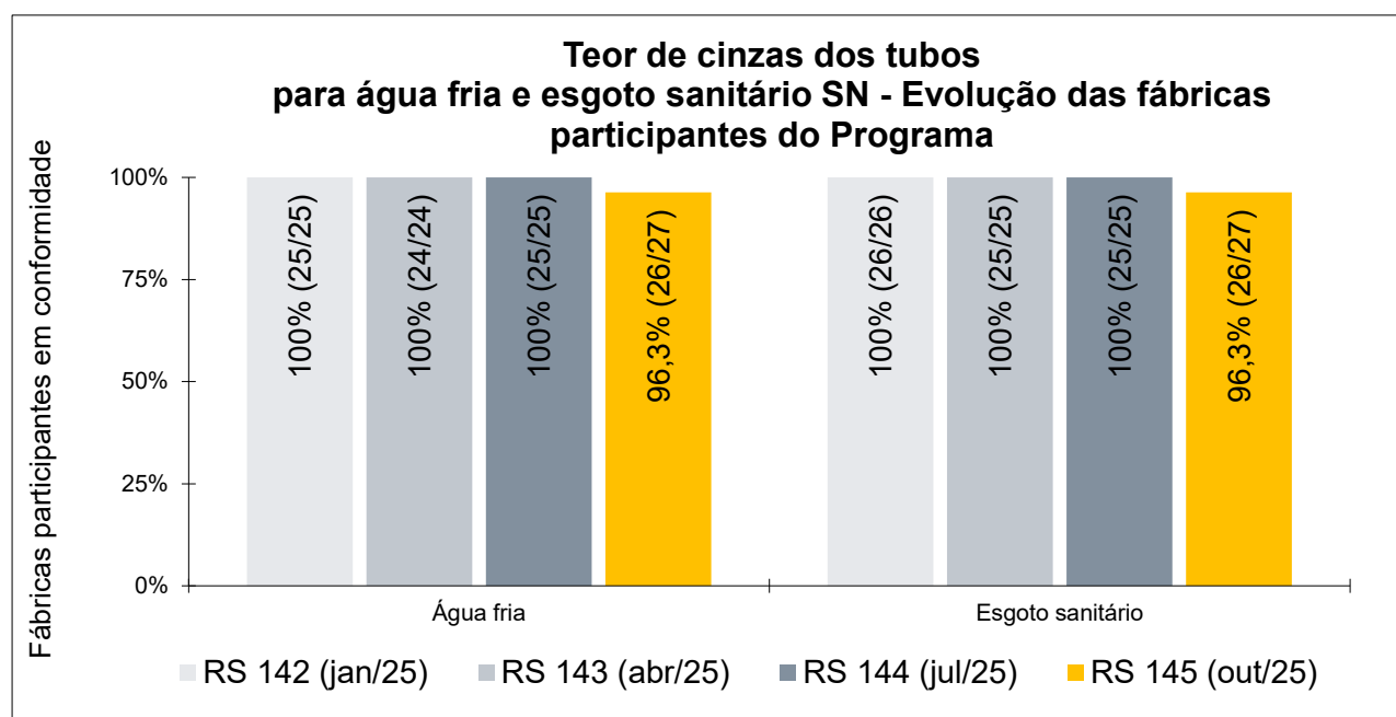
Figura 3 - Teor de cinzas do composto dos tubos para água fria e esgoto sanitário SN
