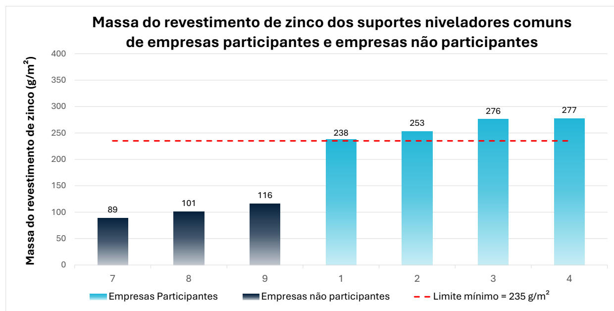
Figura 22 – Resultados da determinação da massa de revestimento de zinco das amostras de suporte nivelador comum avaliadas de empresas participantes e empresas não participantes (o resultado refere-se à média aritmética da massa de zinco de três suportes da mesma amostra)
