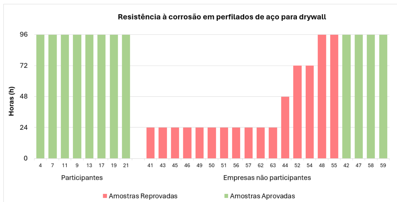
Figura 15 – Resultados da determinação da resistência à corrosão das amostras de perfilados de aço de empresas participantes e não participantes avaliadas
