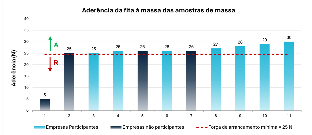
Figura 24 – Resultados da verificação da aderência da fita à massa das amostras de massa para tratamento de juntas avaliadas (empresas participantes e não participantes)
