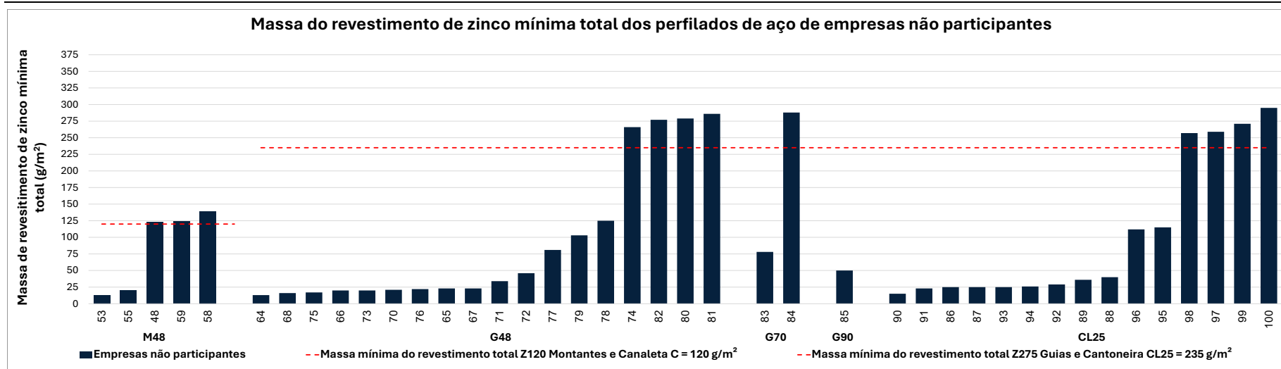
Figura 21 – Resultados da determinação da massa do revestimento de zinco total (nas duas faces) das amostras de perfilados de aço de empresas não participantes avaliadas
