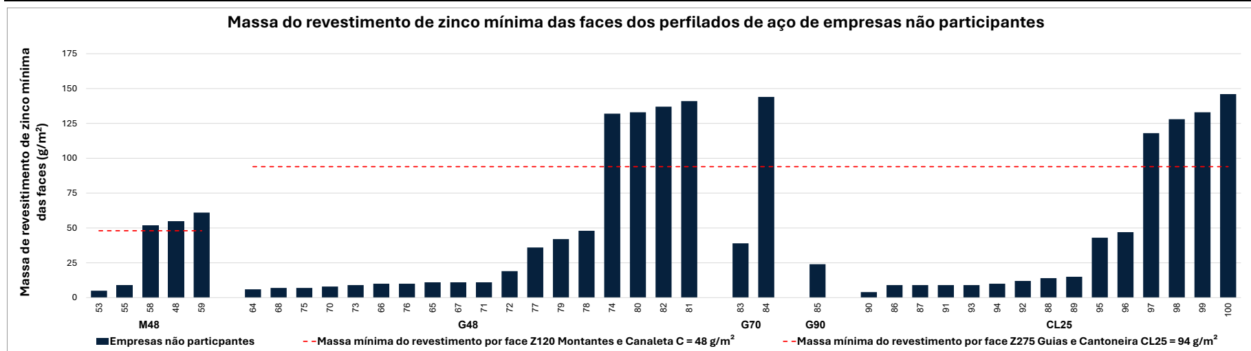
Figura 20 – Resultados da determinação da massa do revestimento de zinco mínima das faces das amostras de perfilados de aço de empresas não participantes avaliadas
