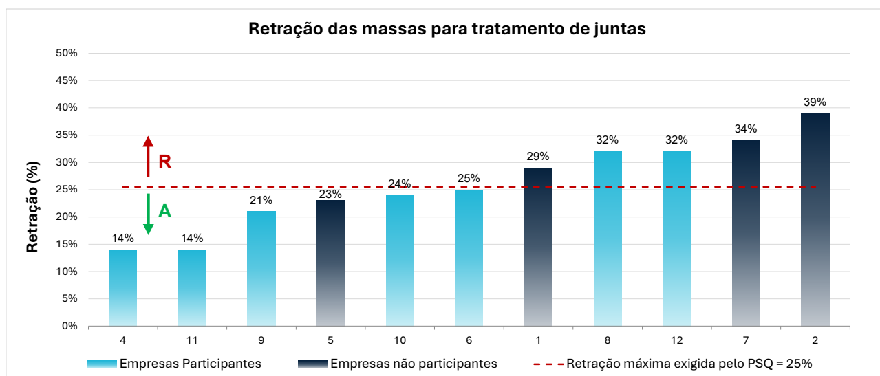
Figura 25 – Resultados da verificação da retração das amostras de massa para tratamento de juntas avaliadas (empresas participantes e não participantes)
