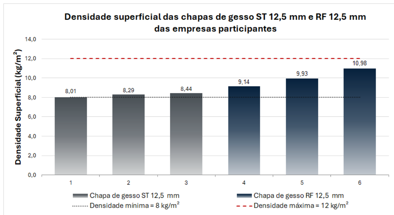
Figura 12 – Resultados da determinação da densidade superficial das amostras de chapas de gesso ST 12,5 mm e RF 12,5 mm
