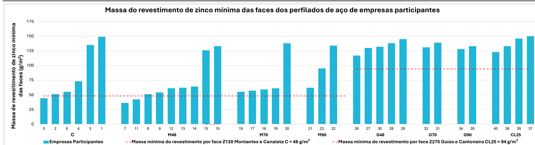
Figura 18 – Resultados da determinação da massa do revestimento de zinco mínima das faces das amostras de perfilados de aço de empresas participantes avaliadas
