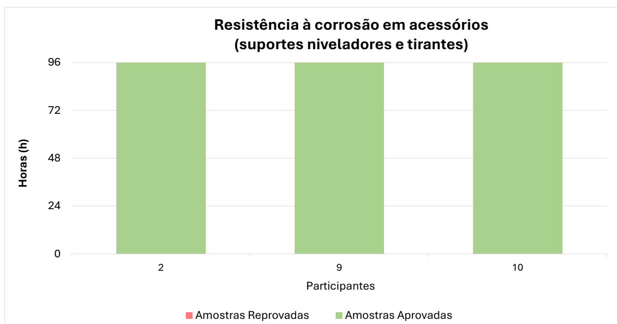
Figura 23 – Resultados da determinação da resistência à corrosão das amostras de suporte nivelador comum e tirantes avaliadas de empresas participantes
