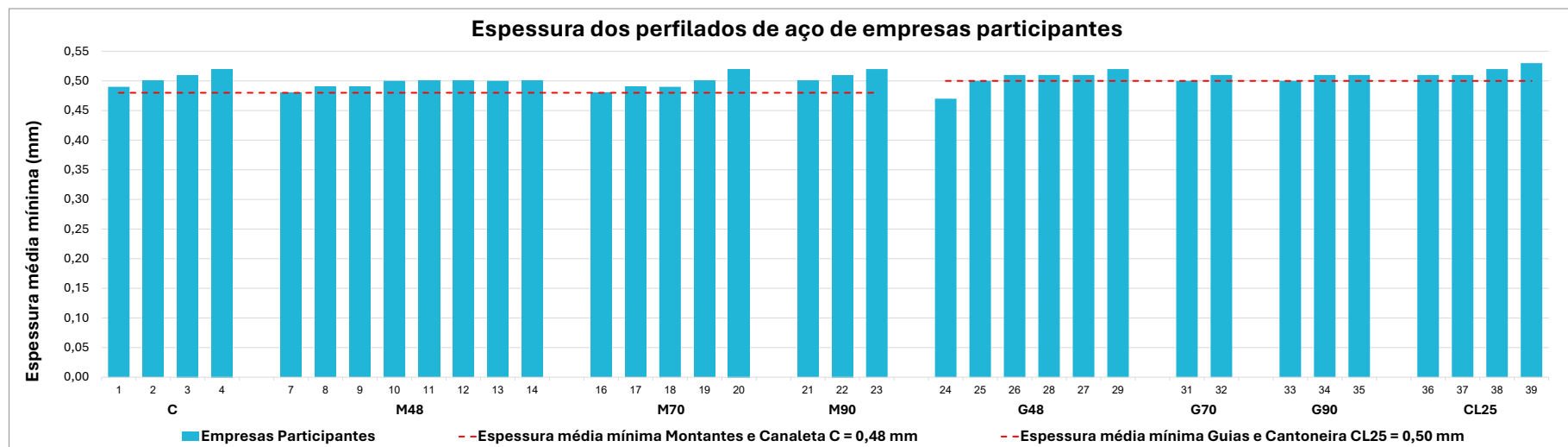
Figura 16 – Resultados da determinação da espessura das amostras de perfilados de aço de empresas participantes avaliadas
