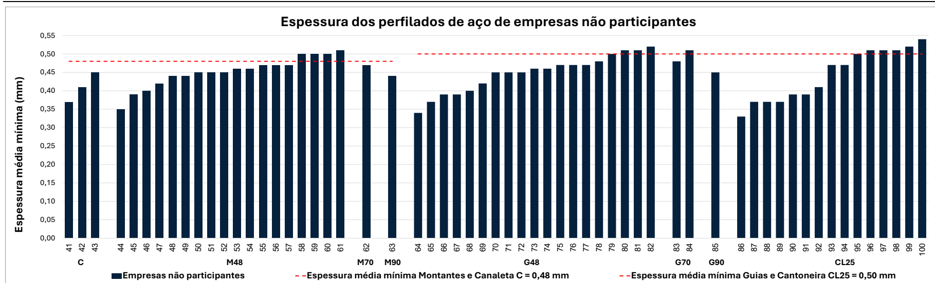
Figura 17 – Resultados da determinação da espeSSura das amostras de perfilados de aço de empresas não participantes avaliadas
