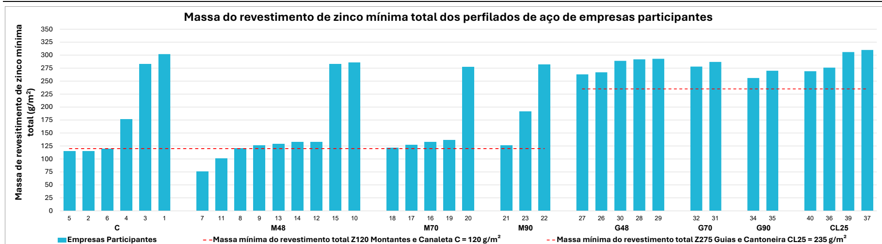
Figura 19 – Resultados da determinação da massa do revestimento de zinco total (nas duas faces) das amostras de perfilados de aço de empresas participantes avaliadas
