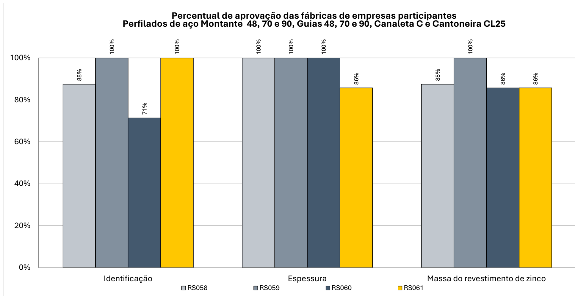
Figura 27 – Percentual de aprovação das fábricas de empresas participantes fabricantes de perfilados de aço
