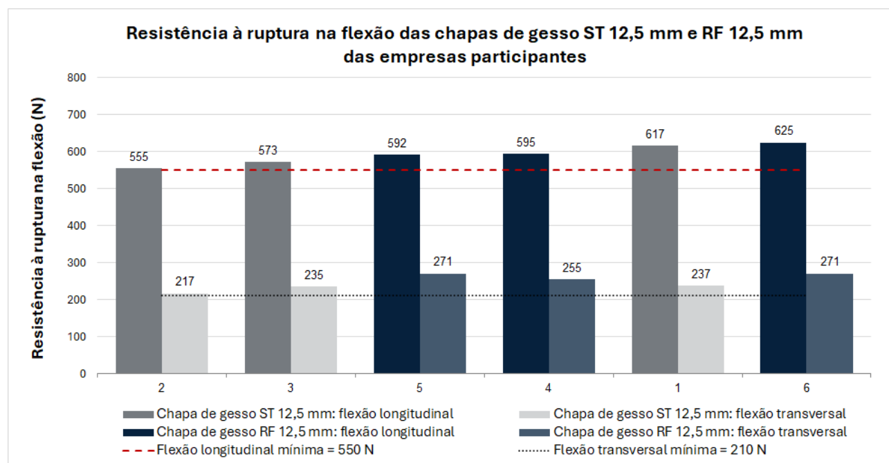
Figura 13 – Resultados da determinação da resistência à flexão (média) das amostras de chapas de gesso ST 12,5 mm e RF 12,5 mm avaliadas
